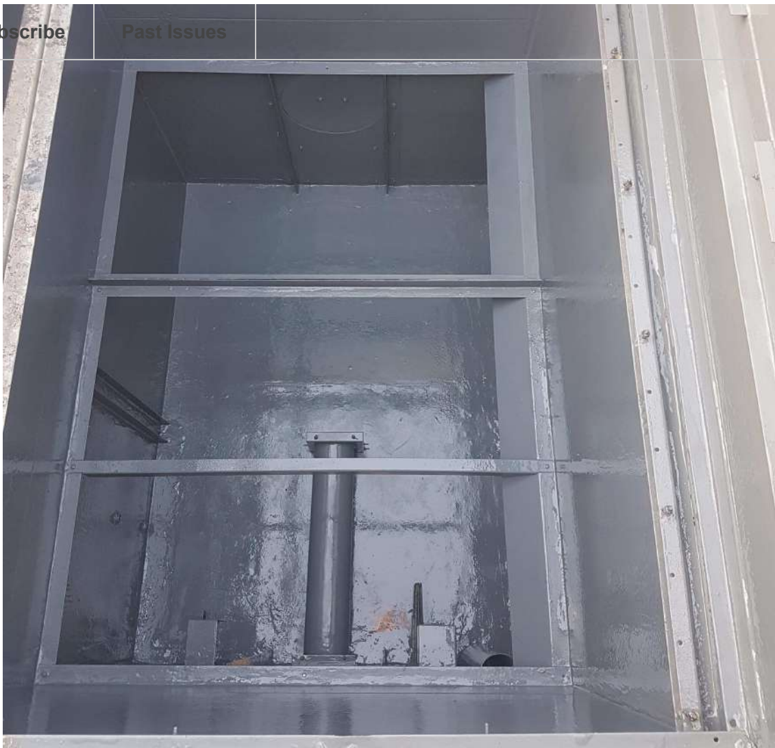
Réfection de l'intérieur d'une tour aéroréfrigérante
